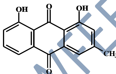
Chrysophanol
