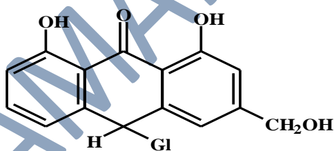
Barbaloin
