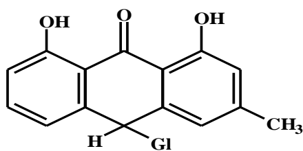
Chrysaloin
