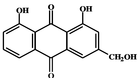
Aloe emodin
