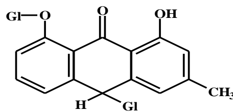
Cascaroside C & D
