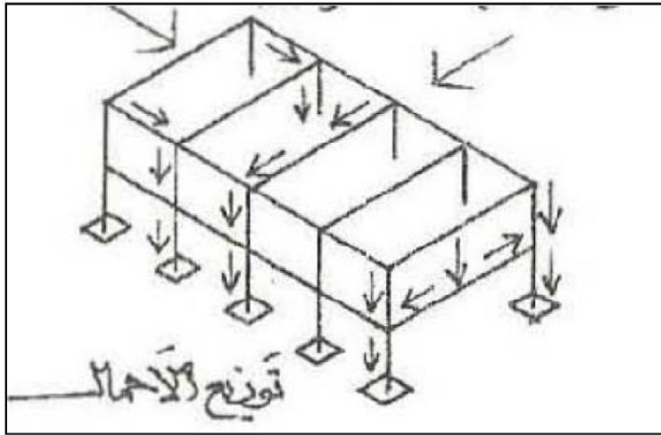
٣- توزيع الاحمال
