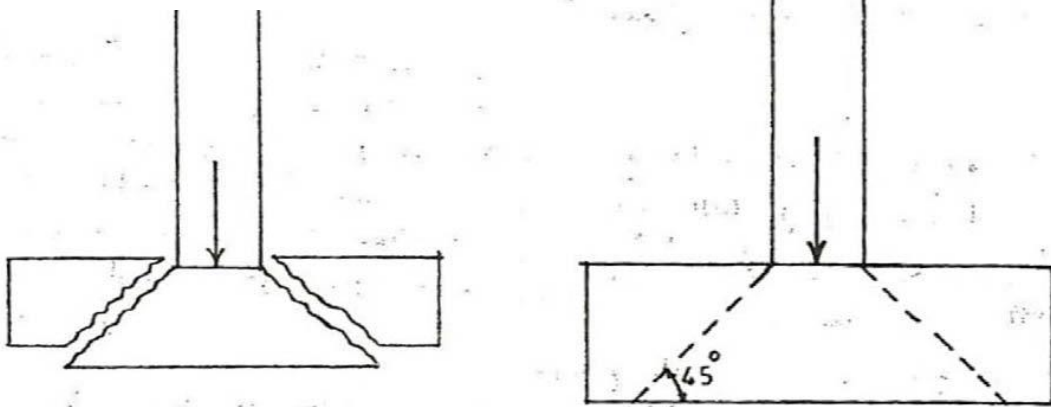
الشكل رقم (٥) الفشل بسبب القص القطري في الاساس الجداري
