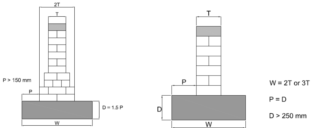
الشكل رقم (٦) عرض الاساس المستمر
