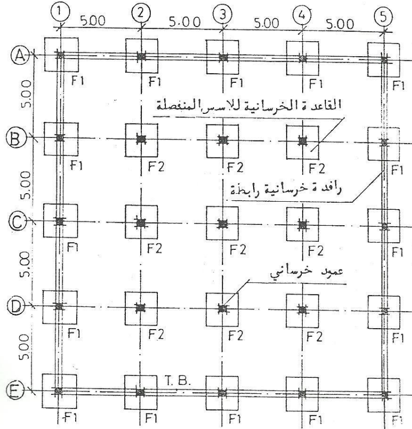
الشكل رقم (٢) الاس المنفصلة
