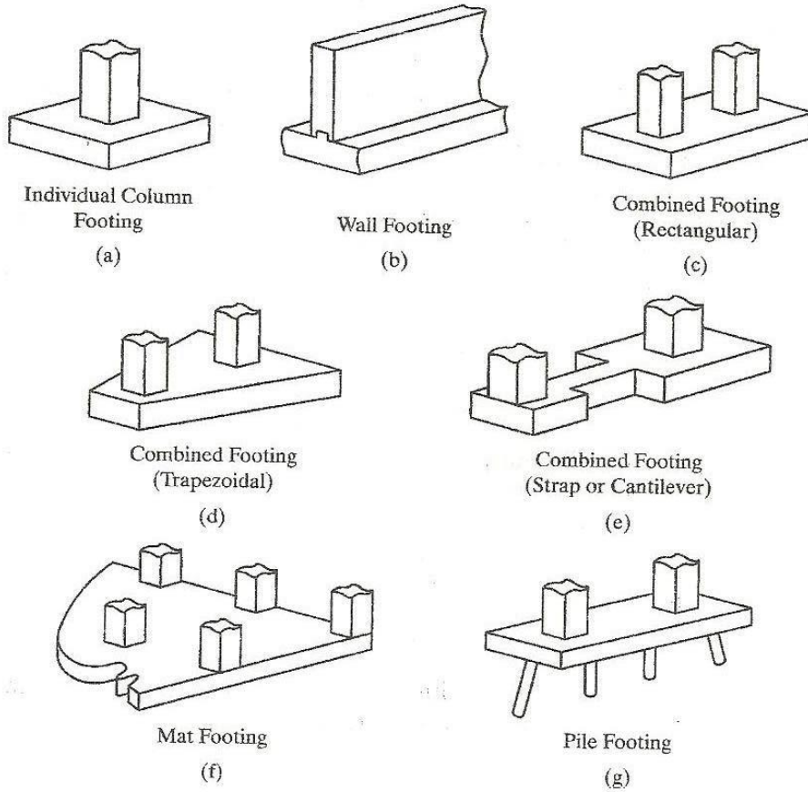
الشكل رقم (١) أنواع الأسس
