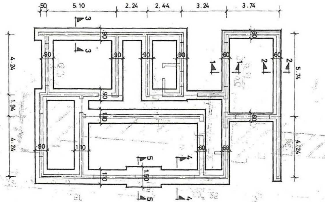
الشكل رقم (٤) الاساس المستمر (الاساس الجداري)
