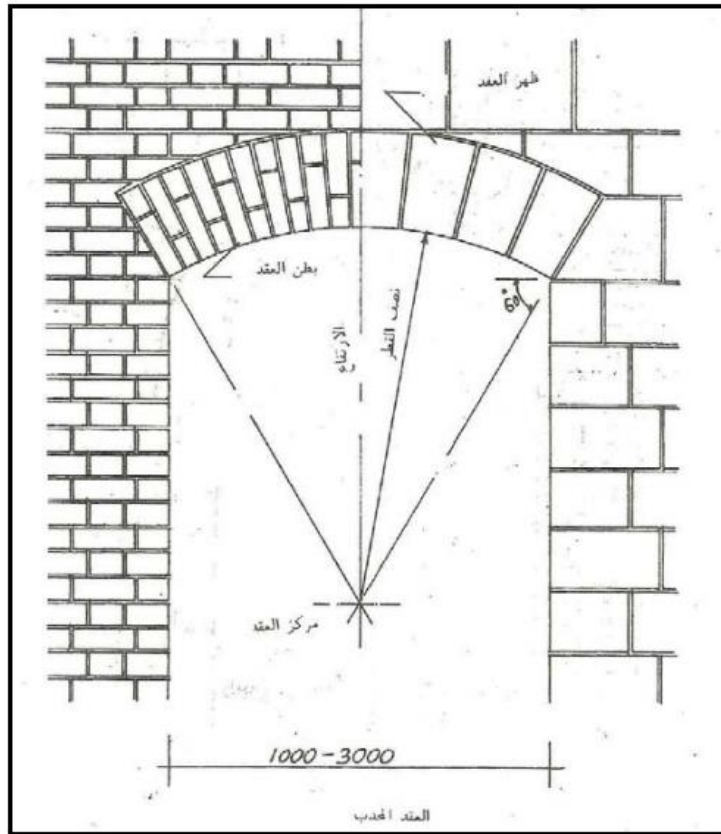
الشكل رقم (8) العقد الهلالي
