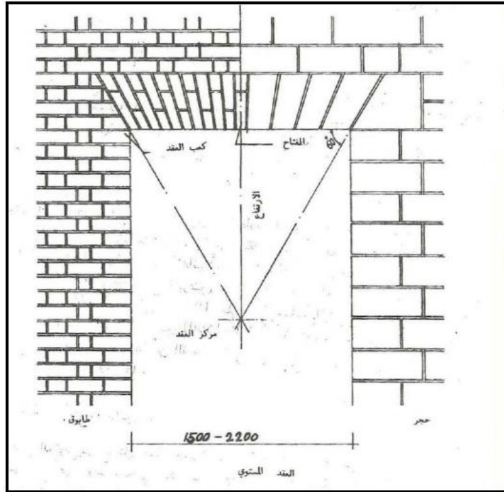
الشكل رقم (5) العقد المستقيم
