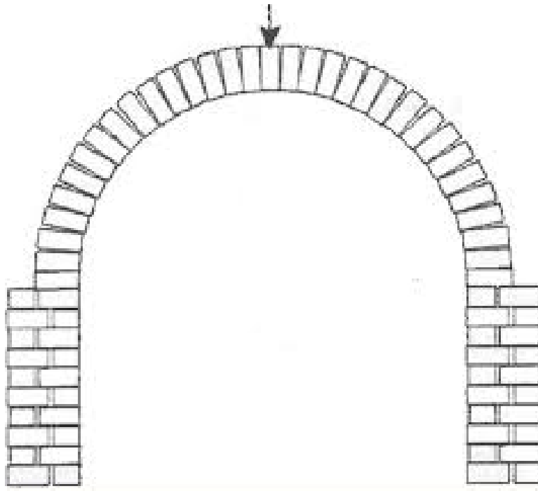
الشكل رقم (4) اصطلاحات العقود
