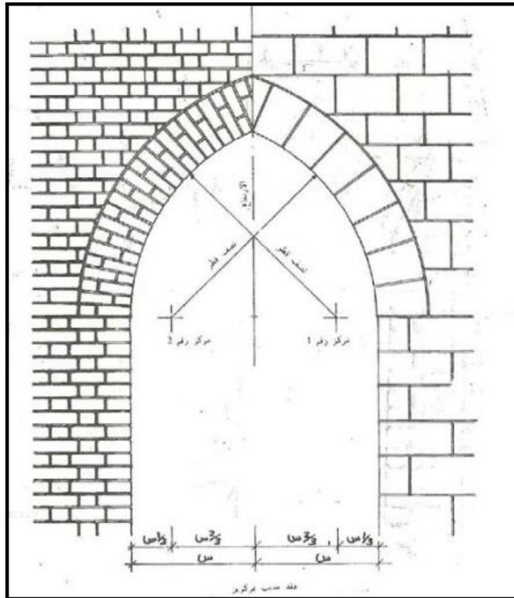
الشكل رقم (7) العقد الدائري
