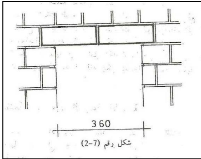
الشكل رقم (2) فتحة بعرض (360 ملم)
