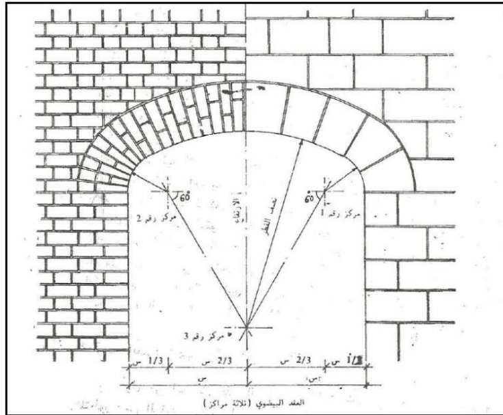
الشكل رقم (9) العقد البيضوي
