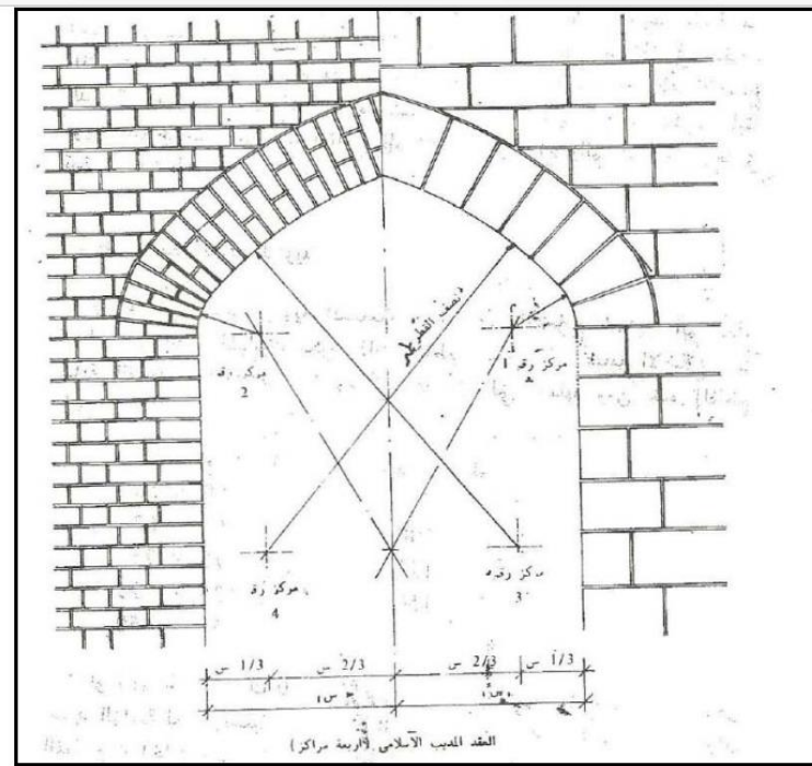
الشكل رقم (10) العقد المدبب ذو الأربعة مراكز
