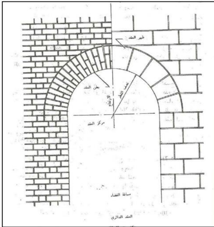
الشكل رقم (6) العقد الدائري
