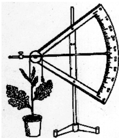
Fig. 5.25 Lever auxanometer
