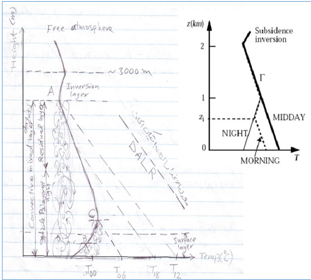
الشكل (3-11): يبيّن تغيّار درجة الحرارة مع الارتفاع خلال النهار والليل مع تحديد ارتفاع الخط.
