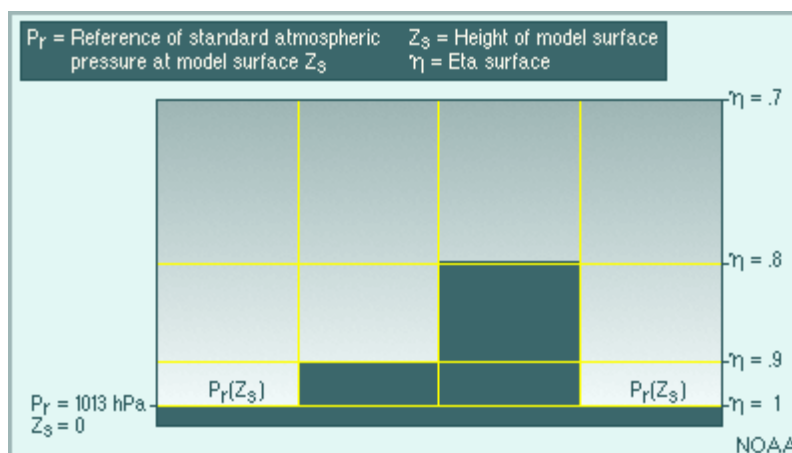
Figure (17.2) Eta vertical coordinate
