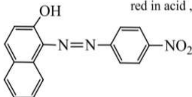
P-nitro azo-2-naphthol para red
